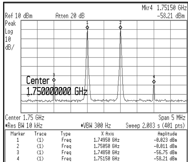
OIP3
